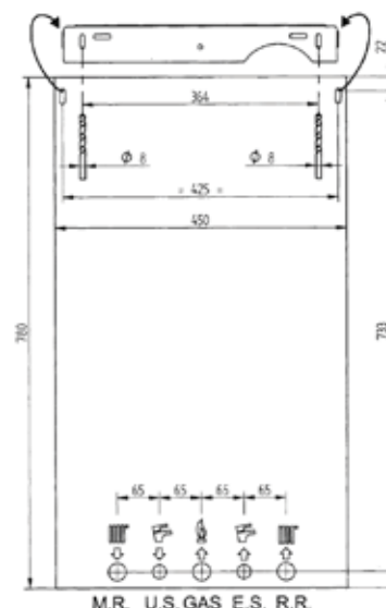
Dima di montaggio
