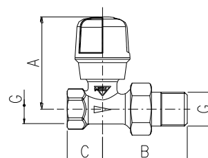
DIRITTA per KIT cod. 2083
