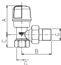
ANGOLO per KIT cod. 2082
