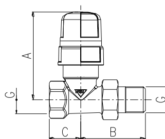
DIRITTA per KIT cod. 2079-2081
