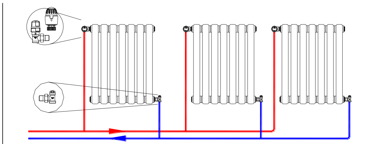
Figura 1 – Composizione tipo impianto di riscaldamento:
