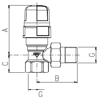
ANGOLO per KIT cod. 2078-2080
